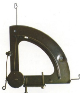
CWN-M673 MULLER鉤邊機 緯紗張力器
