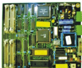
CWN-M033 MULLER III 龍頭介面電子板 179 739 156
