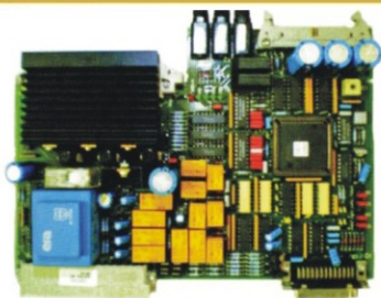
CWN-M029 MULLER III 電流電子板 179 729 188
