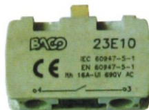
CWN-M051 開關 BACO 23E10
